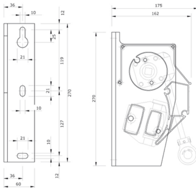
Vooraanzicht muursteun links
