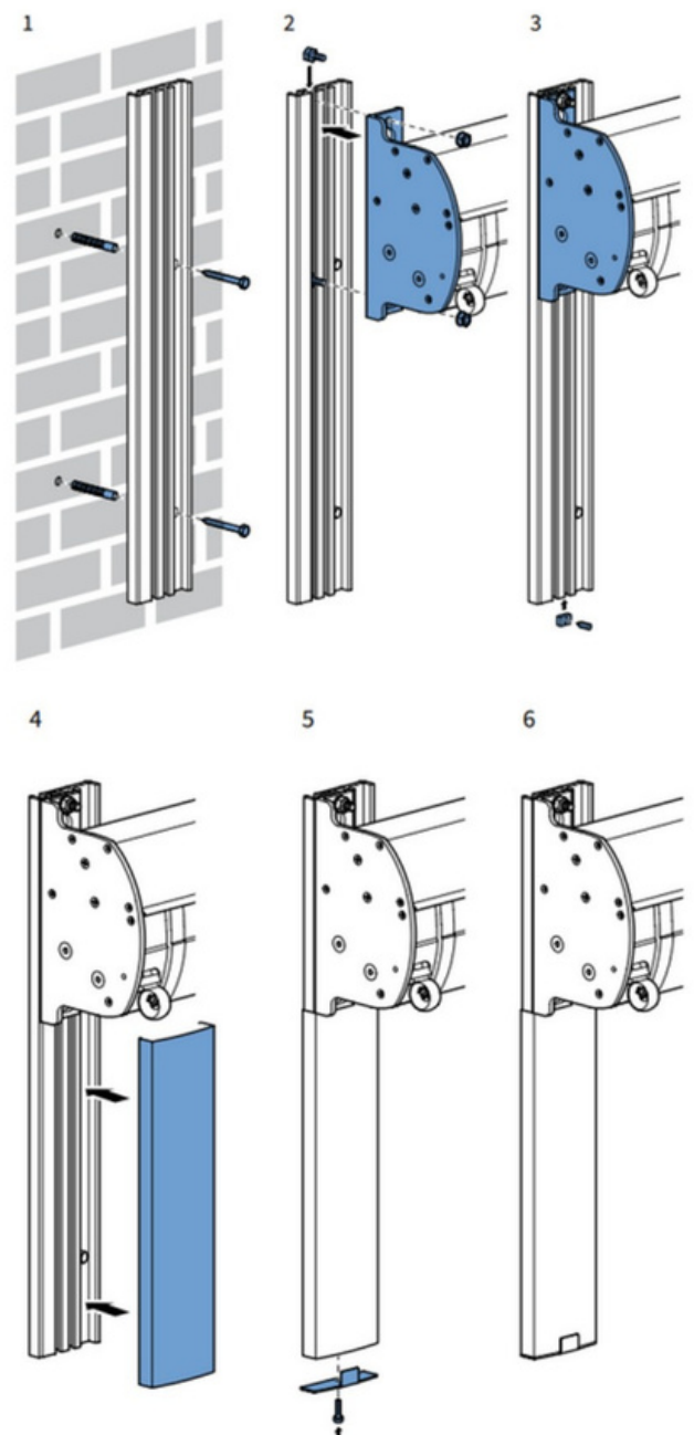
Fig. 1.4 montage van muurstrips (links)
