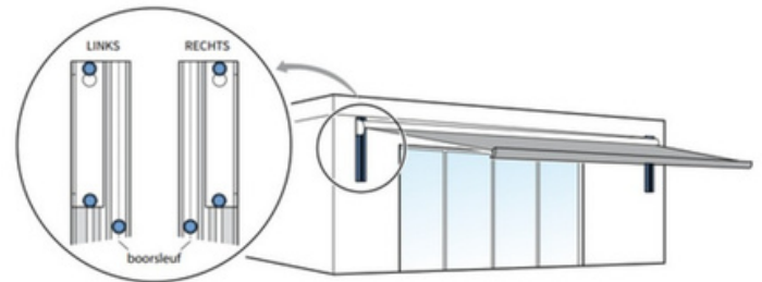
Fig. 1.3 muursteunen knikarmscherm
