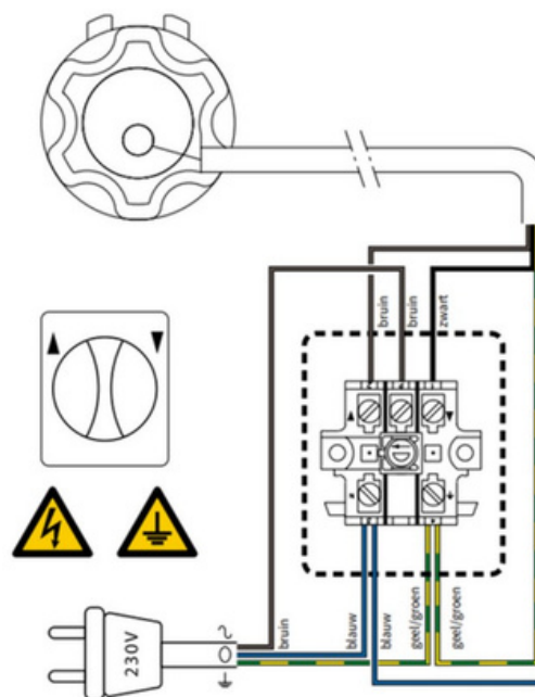
Fig. 2.1 motor links (van buitenaf gezien)
