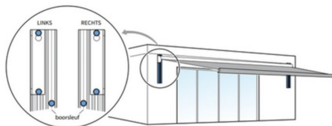
Fig. 1.3 muursteunen knikarmscherm
