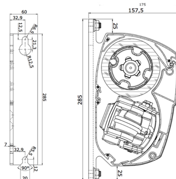
Vooraanzicht muursteun links
