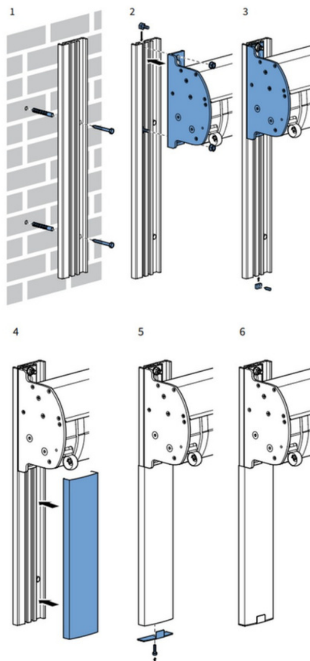
Fig. 1.4 montage van muurstrips (links)
