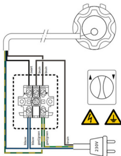
Fig. 2.2 motor rechts (van buitenaf gezien)
