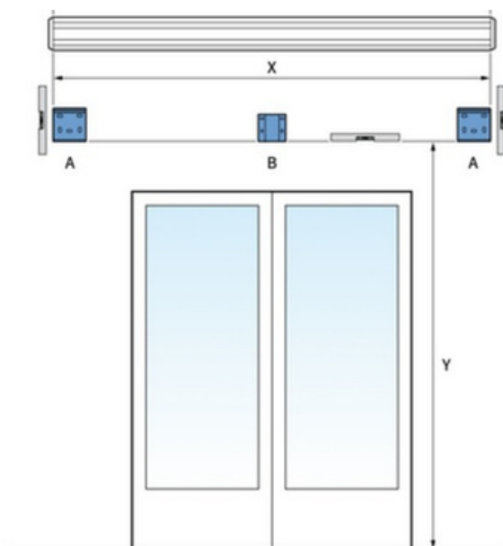
Fig. 1.1 plaatsing muurstenen
