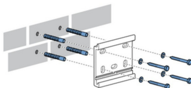
Fig. 1.2 monteren muurstenen
