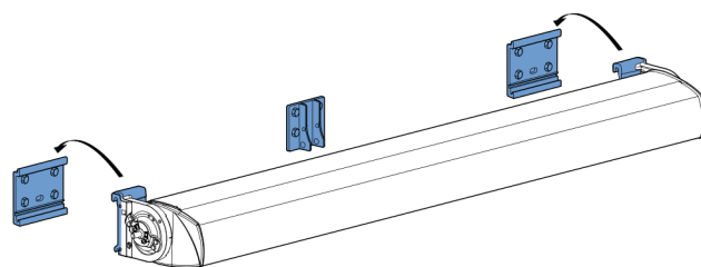
Fig. 2.1 Ophangen scherm
