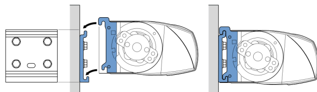
Fig. 2.2 Detail muursteun A
