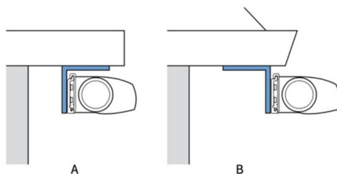
Fig. 9.2 Toepassing van plafondbeugels
