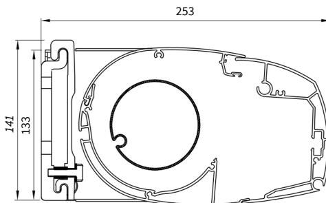
zijaanzicht scherm
