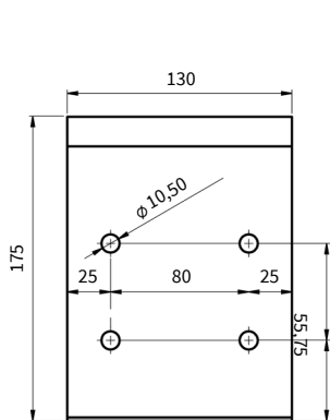
vooraanzicht plafondsteun
