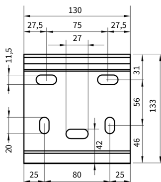
vooraanzicht muursteun
