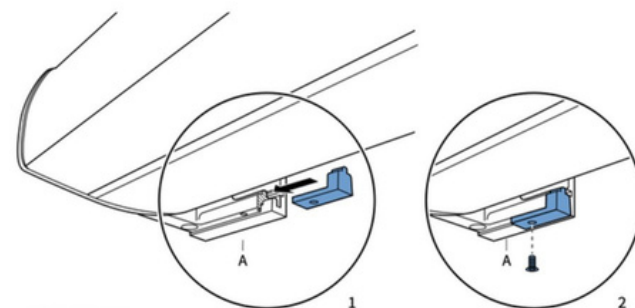
Fig. 2.4 Detail borgblokje
