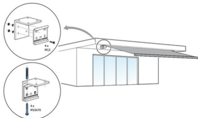
Fig. 9.1 Plafondmontage
