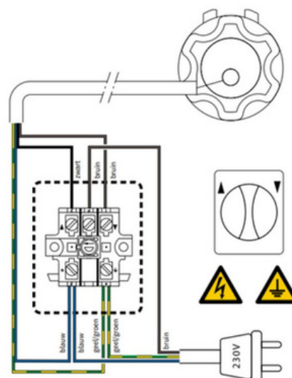
Fig. 3.2 motor rechts (van buitenaf gezien)
