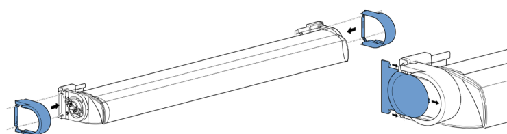
Fig. 7.1 Motoren zijkappen
