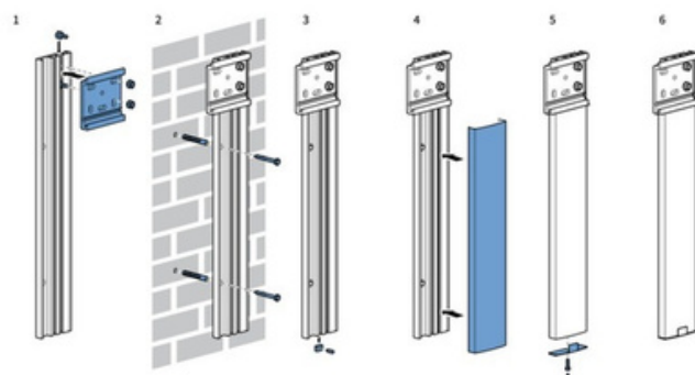
Fig. 8.2 Montage van muurstrips rechts
