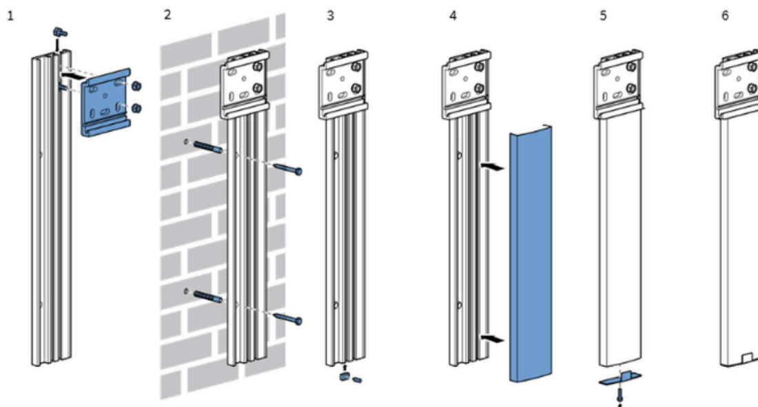
fig. 8.2 Montage van muurstrip rechts
