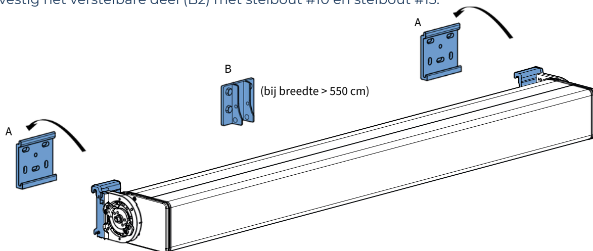
fig. 2.1 Ophangen scherm
