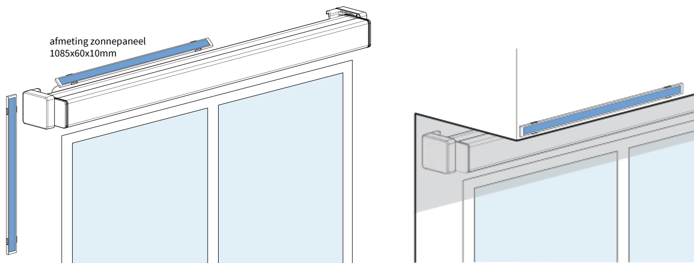
fig. 5.1 Positionering zonnepaneel
