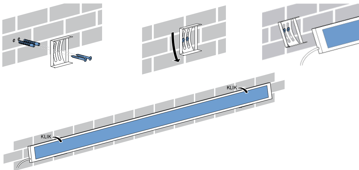
fig. 5.2 Montage zonnepaneel
