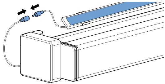
fig. 5.3 Aansluiten zonnepaneel
