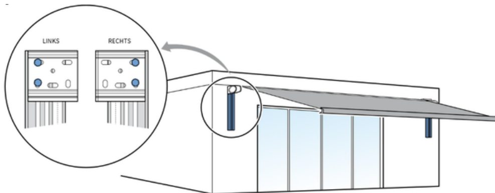
fig. 8.1 Toepassing van muurstrips
