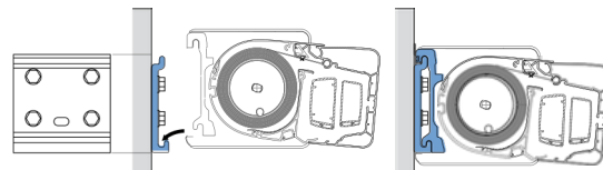
Fig. 2.2 Detail muursteun A
