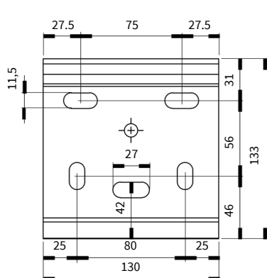
vooraanzicht muursteun
