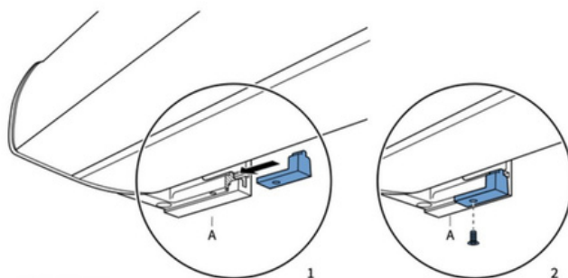
Fig. 2.4 Detail borgblokje
