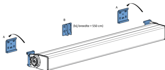
Fig. 2.1 Ophangen scherm
