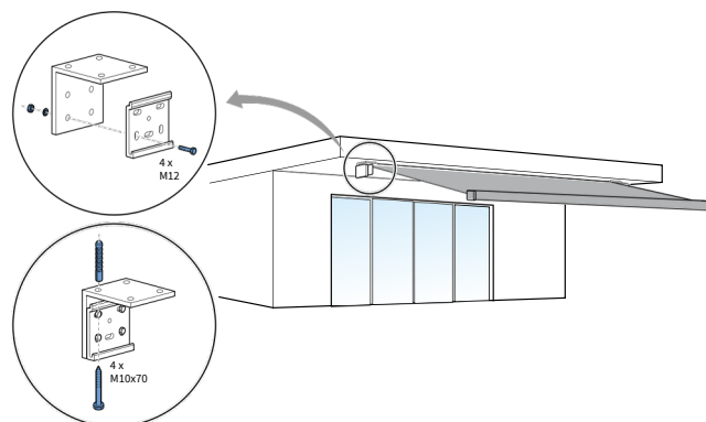
Fig. 7.1 Plafondmontage
