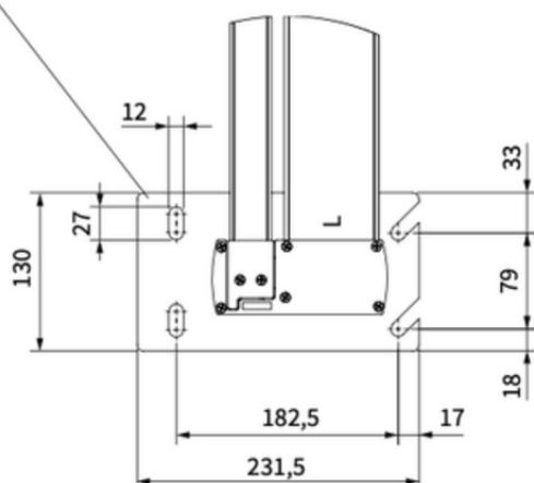
Balkonvoet zijvleugel rechtsachter WC.745.00.01.31
