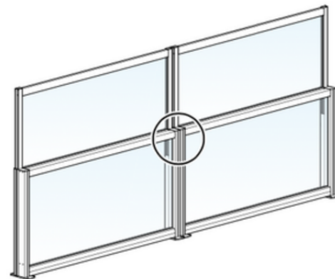
fig. 3.1 Locatie koppeling
