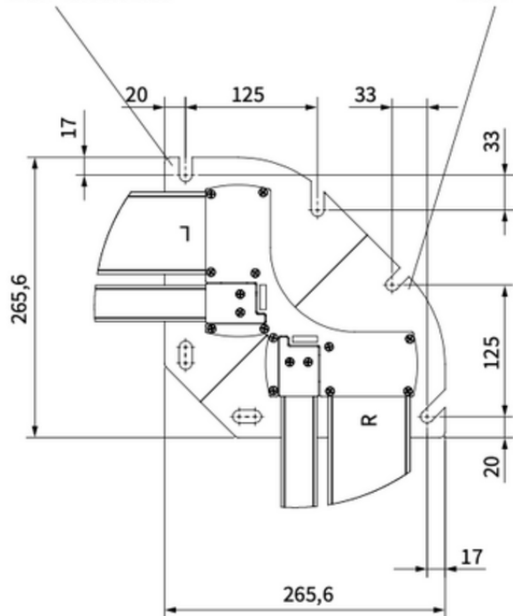
Balkonvoet rechtsvoor WC.745.00.01.35
