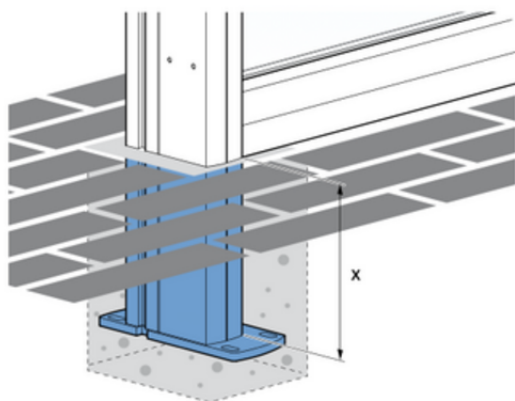
fig. 2.1 Verzonken voetplaat
