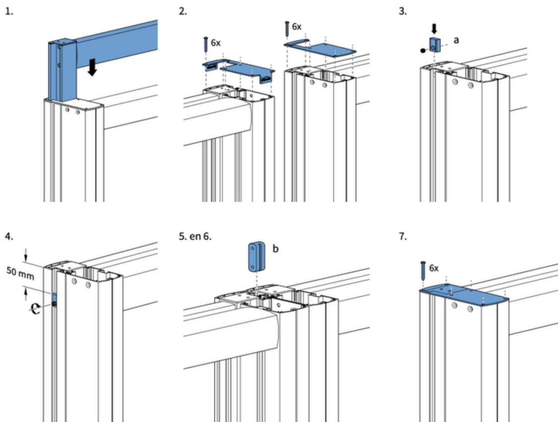
fig. 3.2 Montage koppeling
