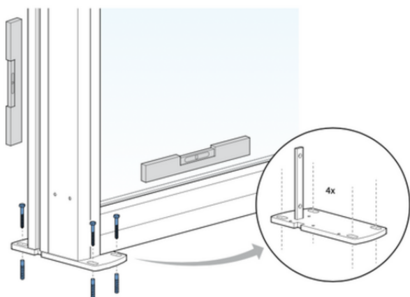
fig. 1.2 Vastschroeven voetplaat
