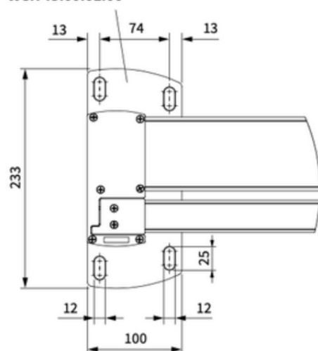
Bevestigingsvoet standaard links WC.745.00.01.00
