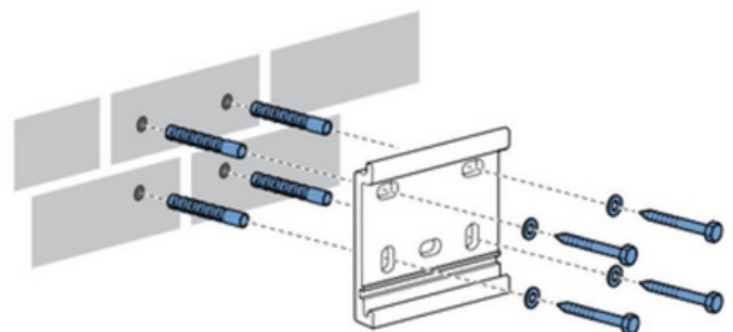
Fig. 1.2 monteren muurstenen
