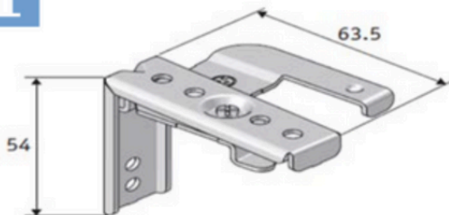
Beugel 35 - 50 - 70 mm
