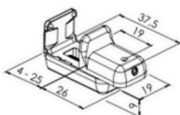
Klemsteun draai/kiepraam 25 mm onderkant
