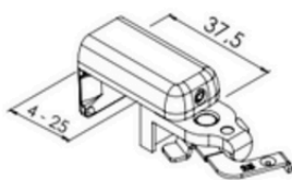
Klemsteun draai/kiepraam 25 mm bovenbak - bovenkant
