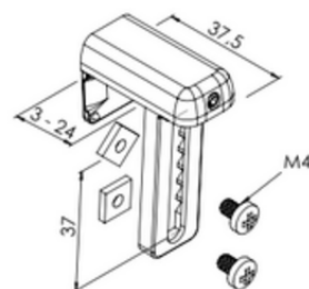
Klemsteun draai/kiepraam 50 mm bovenbak - bovenkant
