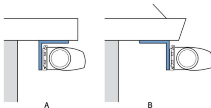
fig. 9.2 Toepassing van plafondbeugels
