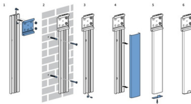
fig. 8.2 Montage van muurstrip rechts
