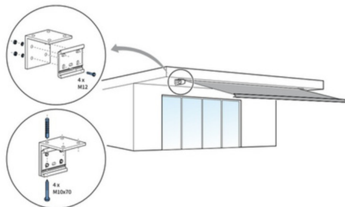
figuur 9.1 Plafondmontage
