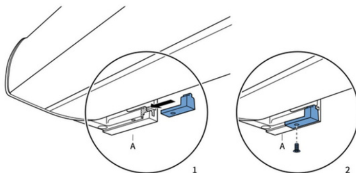
fig. 2.4 Detail borgblokje
