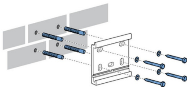
fig. 1.2 Monteren muursteunen
