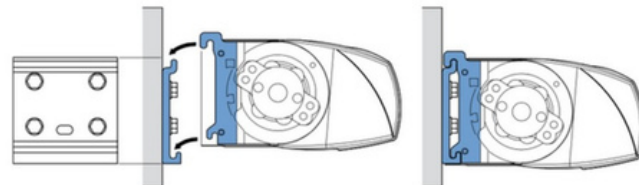
fig. 2.2 Detail muursteun A
