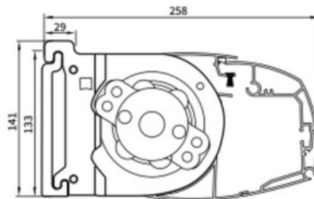
schermdoorsnede
