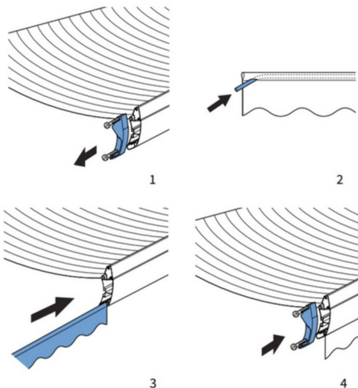
Fig. 6.1 plaatsen volant
