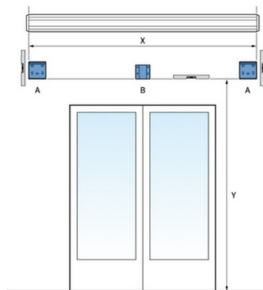
fig. 1.1 Plaatsing muursteunen
