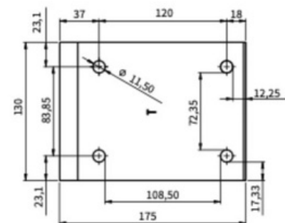
bovenaanzicht plafondsteun
