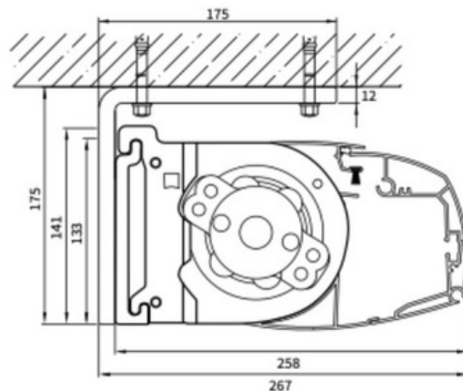
schermdoorsnede
