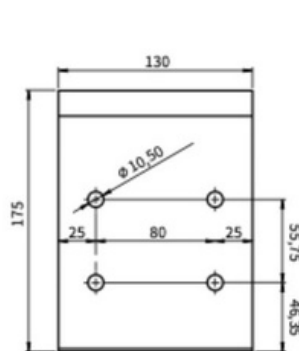
vooraanzicht plafondsteun
