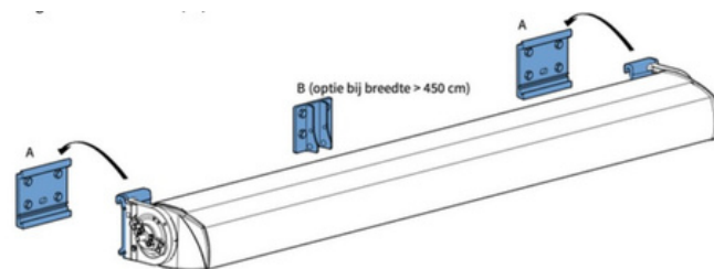
fig. 2.1 Ophangen scherm
