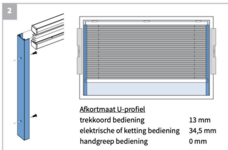
C 'op de dag' montage met afstandsteun
