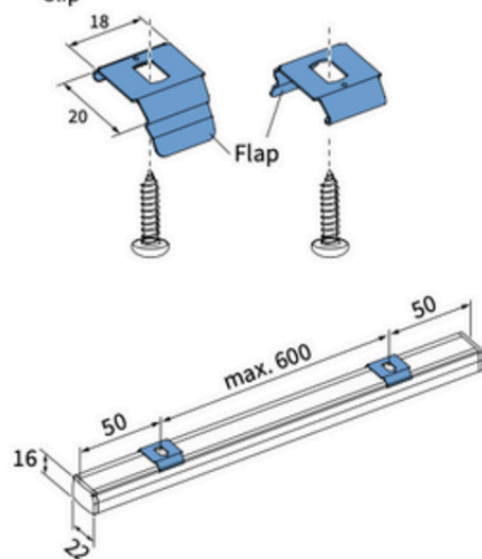
Standaard profiel 40 Clip
