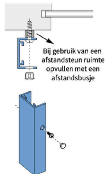
C 'op de dag' montage met afstandsteun
