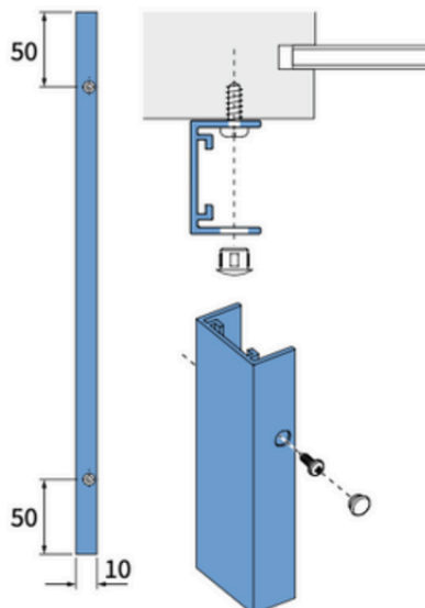
B 'op de dag' montage
