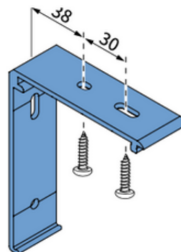
Plafondmontage
